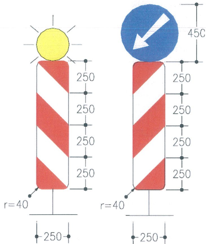
Εικόνα 7 – Διαστάσεις πινακίδων οριοθέτησης διαδρόμου κυκλοφορίας
