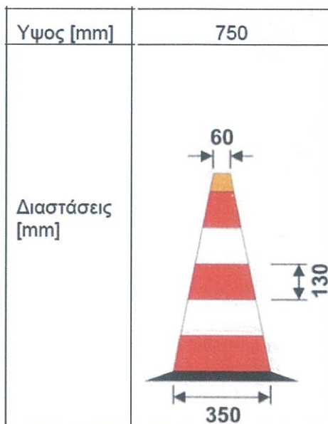
Εικόνα 6 – Διαστάσεις κυκλοφοριακών κώνων
