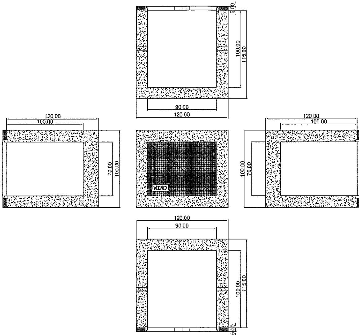
Εικόνα 2 - Φρεάτιο διαστάσεων 90x70cm
