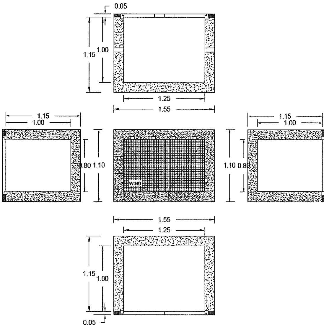
Εικόνα 2 - Φρεάτιο διαστάσεων 125x80cm
